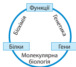
Іл. 89. Предмет досліджень молекулярної генетики
