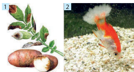
Іл. 26. Несправжні гриби-паразити:
