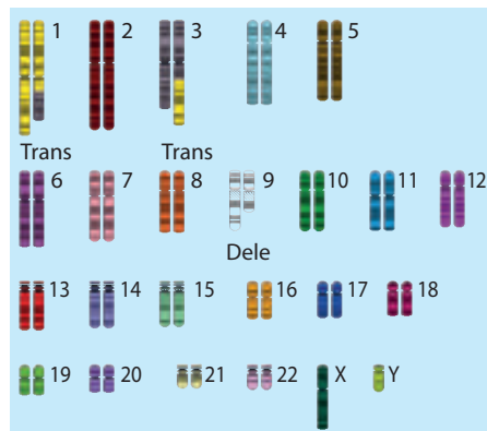
Іл. 97. Хромосомний аналіз кариотипу людини: класичне (з дисками) і спектральне (в кольорі) кариотипування з виявленими хромосомними мутаціями за 1, 3 і 9-тою парами хромосом
