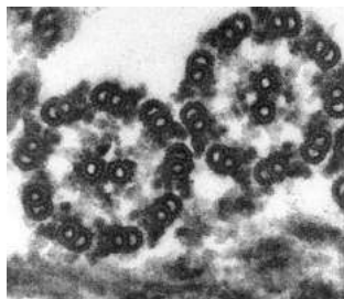
Іл. 21. Поперечний розріз еукаріотичних джгутиків
