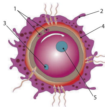
Іл. 137. Запліднений овоцит людини: 1 – полоцити; 2 – променистий вінець; 3 – ядро сперматозоона; 4 – блискуча зона; 5 – ядро овоцита
