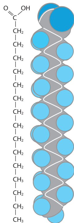
Іл. 59. Пальмітинова кислота ( C_{15}H_{31}COOH ) – насичена жирна кислота
