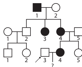
Іл. 105. X-зчеплений домінантний тип успадкування
