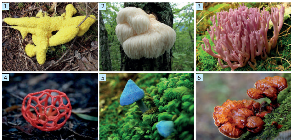
Іл. 24. Незвичні види грибів: 1 – фуліго гнильний; 2 – герацій гребінчастий; 3 – клаварія біло-бура; 4 – решіточник червоний; 5 – ентомола блакитна; 6 – ганодерма блискуча
