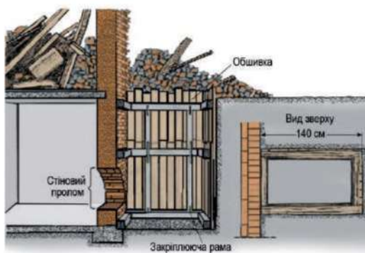
Іл. 35.11. Шахта
