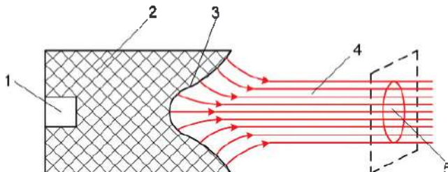
Іл. 3.8. Кумулятивний ефект РКГ-3: 1 — підричник; 2 — заряд; 3 — металева лійка; 4 — гази; 5 — фокус кумуляції (найвузжча частина кумулятивного струменя)
