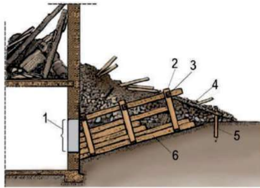
Іл. 34.10. Траншея в уламках: 1 — стіновий пролом; 2 — брус для перекриття; 3 — розтірка; 4 — розкіс; 5 — паля для закріплення; 6 — дошки обшивки
