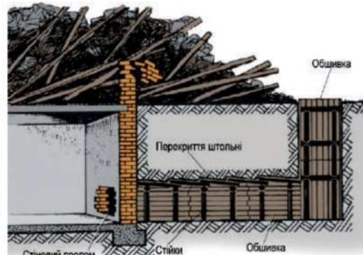
Іл. 34.12. Шахта і штольня
