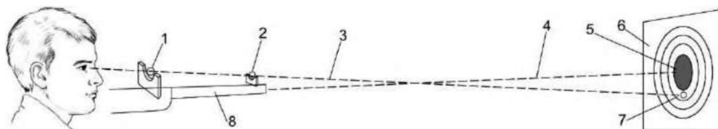
Іл. 2.8. Схема прицілювання в разі перевищення середньої точки прицілювання:
