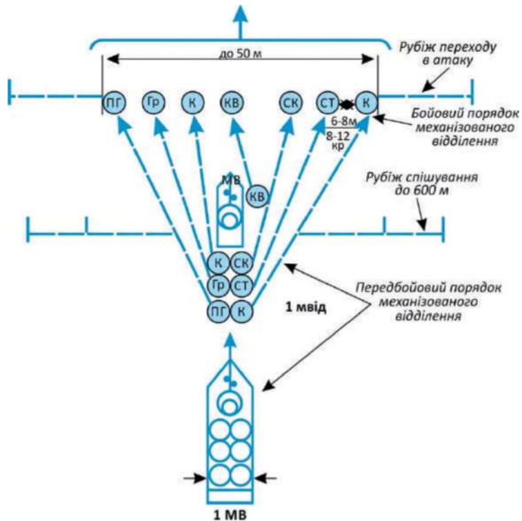
Іл. 13.4. Наступ із висунуттям із глибини (з ходу)
