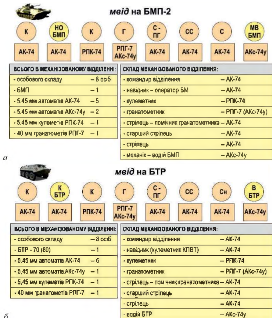
Іл. 6.2. Склад та озброєння механізованого відділення (мвїд) — базового підрозділу для створення бойових груп у ЗСУ: а — на бойовій машині піхоти (БМП); б — на бронетранспортері (БТР)
