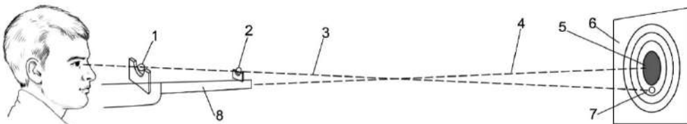
Іл. 21.5 Схема прицілювання в разі перевищення середньої точки прицілювання: 1 — середина прорізу прицілу; 2 — верхній край мушки; 3 — лінія прицілювання; 4 — середня траєкторія кулі; 5 — середня точка влучення — центр мішені; 6 — мішень; 7 — точка прицілювання; 8 — ствол гвинтівки
