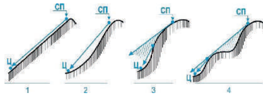
Іл. 33.10. Наявність взаємної видимості точок на одному схилі залежно від форми схилу
