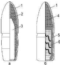
Іл. 22.4. Куля: а — звичайна зі сталевим осердям; б — трасуюча; 1 — оболонка; 2 — свинцева сорочка; 3 — сталевга серцевина; 4 — свинцева серцевина; 5 — стаканчик трасера; б — трасуюча суміш
